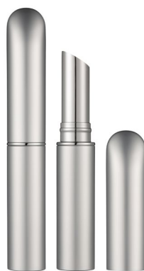
○ HL 8193 SIZE: Φ 14 x 96.5 mm CUP SIZE: Φ 8.5 mm
